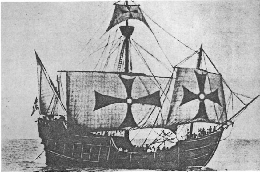
LA "SANTA MARIA" VISTA DE ESTRIBOR (RECONSTRUIDA EN 1929. POR JULIO GUILLEN, CON LINEAS DE CARABELA)
